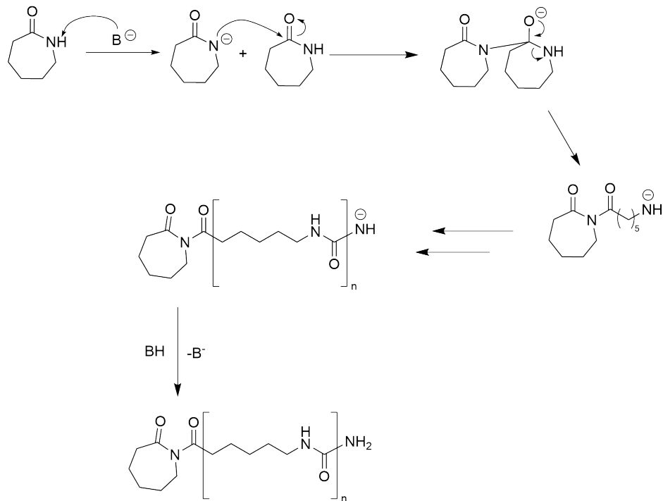
Abb. 7: Die Abbildung zeigt die ringöffnende Polymerisation von \epsilon -Caprolactam zu Nylon-6.
